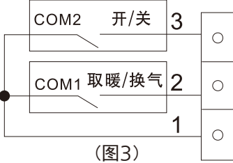
附带2位单控开关接线示意图
