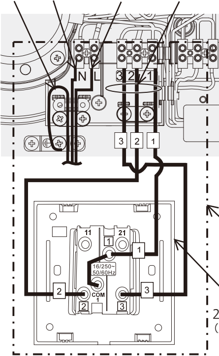
(接线示意图)
