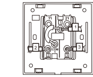
功能开关背面示意图
