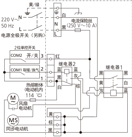
继电器1接线图
